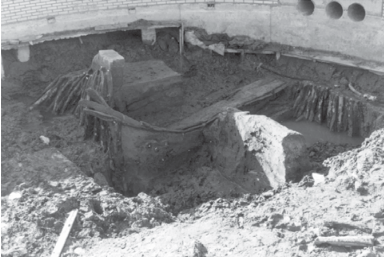
Eén van de Romeinse duikers te Hoogstad, gelegen exact in het verlengde van een moderne duiker die net is aangelegd. Aan weerszijden van de duiker is een dichte paalzetting te zien die tezamen met het aardlichaam ertussen een dam vormde (Foto: Bureau Archeologie en Monumentenzorg, Vlaardingen).
